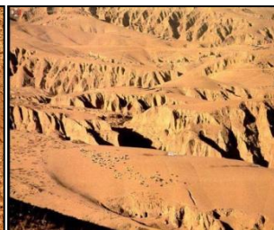
未经治理的黄土高原
