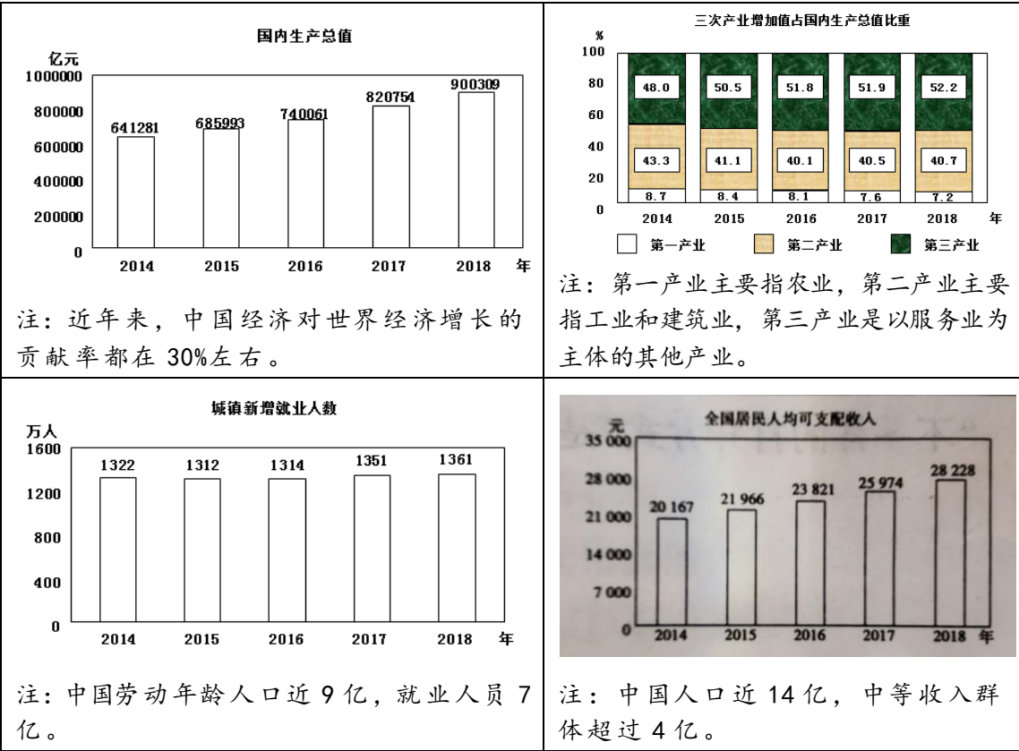
图 12: 近年来我国国民经济与社会发展情况
